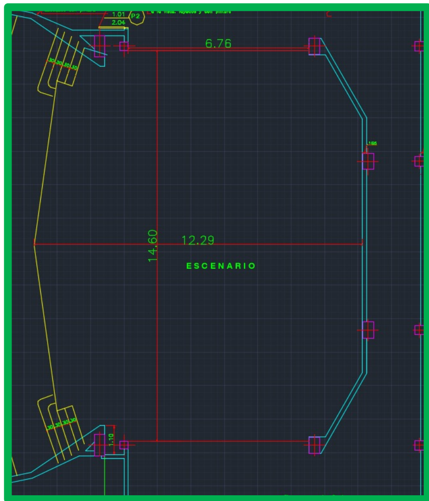
PLANTA
